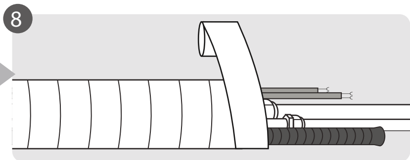
8 Envuelva tuberías y cables (no aplicable para algunos lugares de Norte América)
